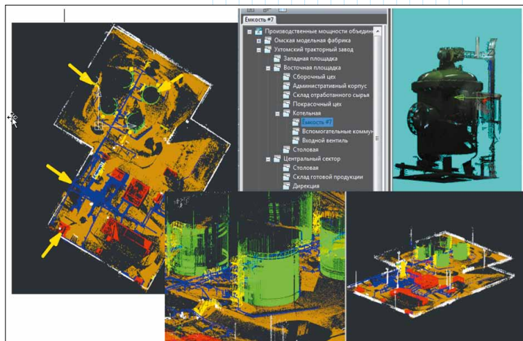
Сегментация
